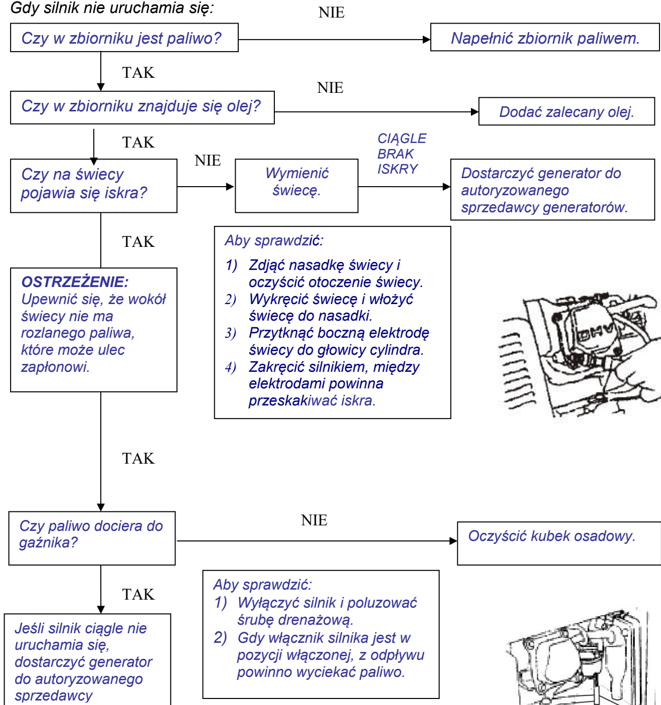
ŚRUBA DRENAŻOWA
